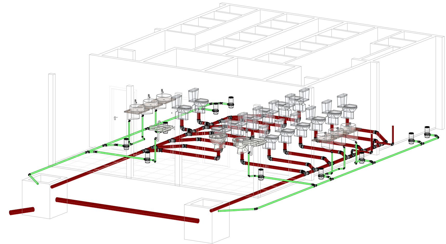
3 VISTA ESG - 3D AA ESCALA -
