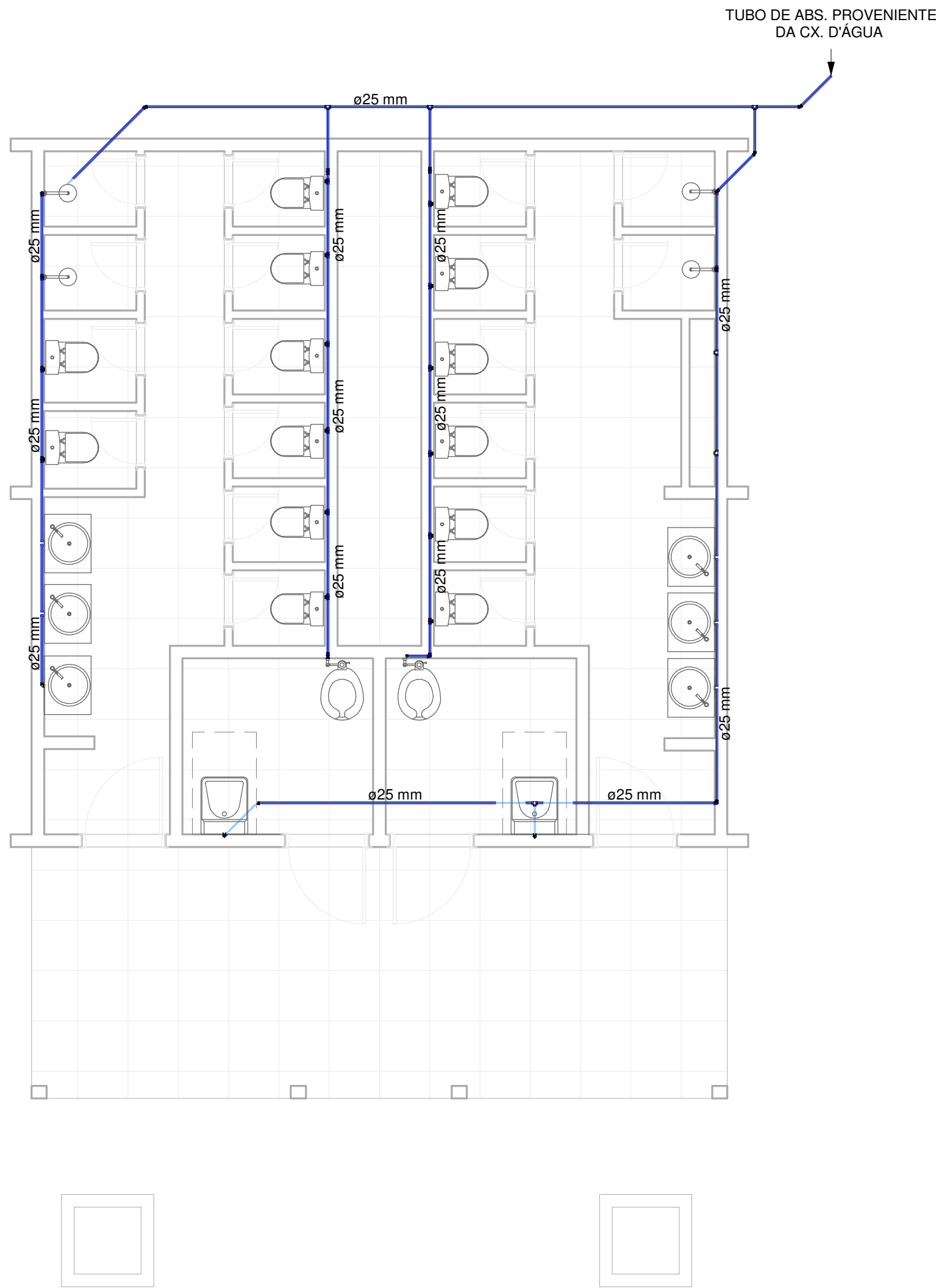
2 ABS - BHO 01 ESCALA - 1 : 50
