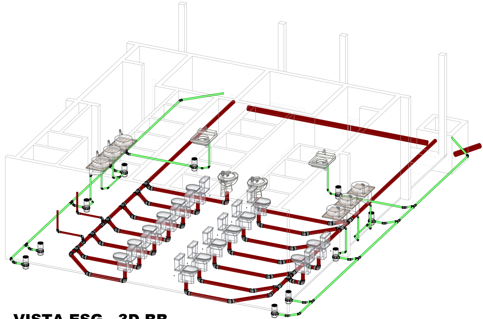
4 VISTA ESG - 3D BB ESCALA -
